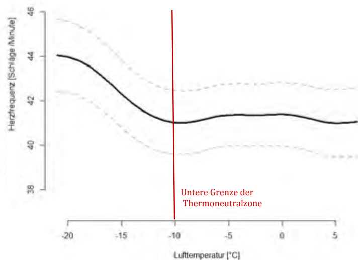
Abb. 3: Veränderung der Herzfrequenz in Abhängigkeit von der Lufttemperatur. Die untere Grenze der Thermoneutralzone liegt bei -10^{\circ}\text{C} , darunter stieg die Herzfrequenz stetig an.
